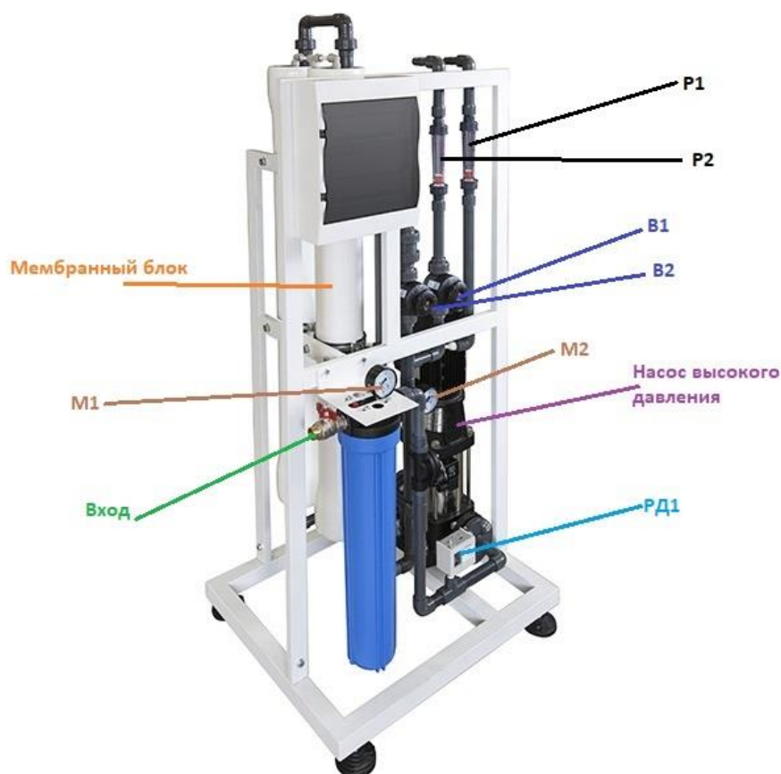
Рис.1 Общий вид установки.
