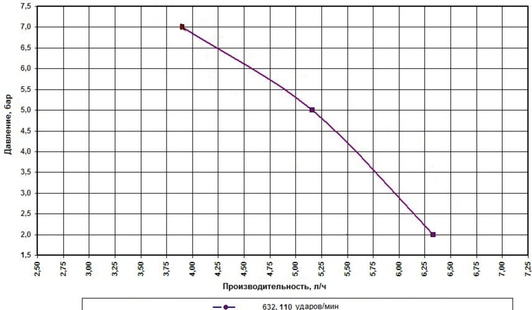
График зависимости производительности насоса
